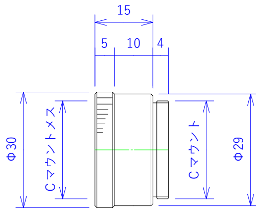
Cマウント接写バレル 15mm AS-EXT15
