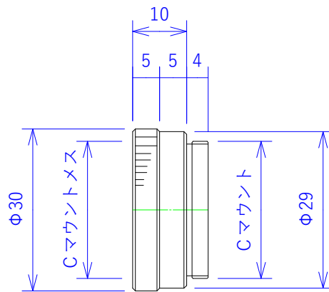
Cマウント接写バレル 10mm AS-EXT10
